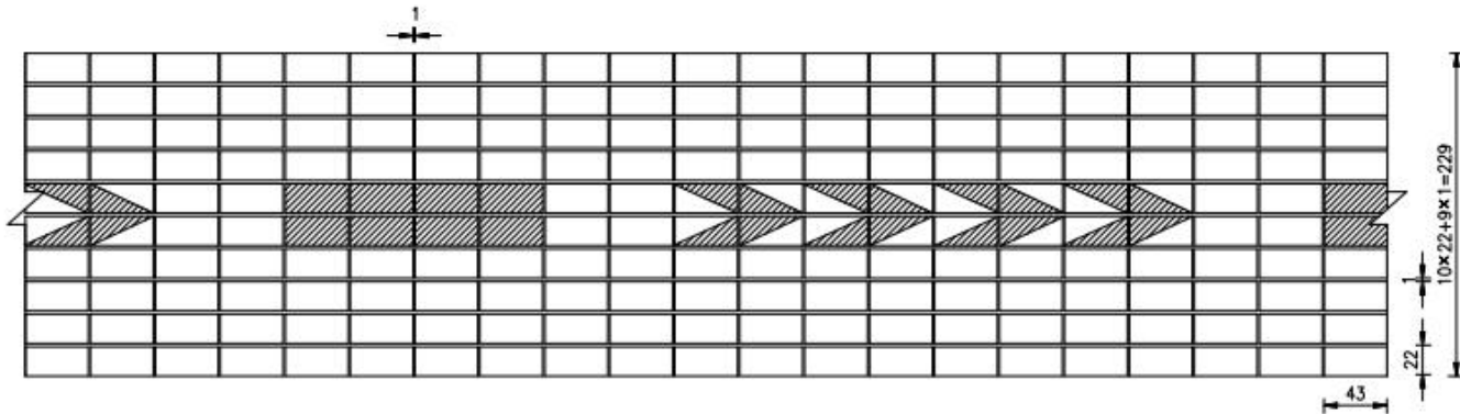
图 6.3-35 边墙隧道专用瓷砖恢复设计展开图
