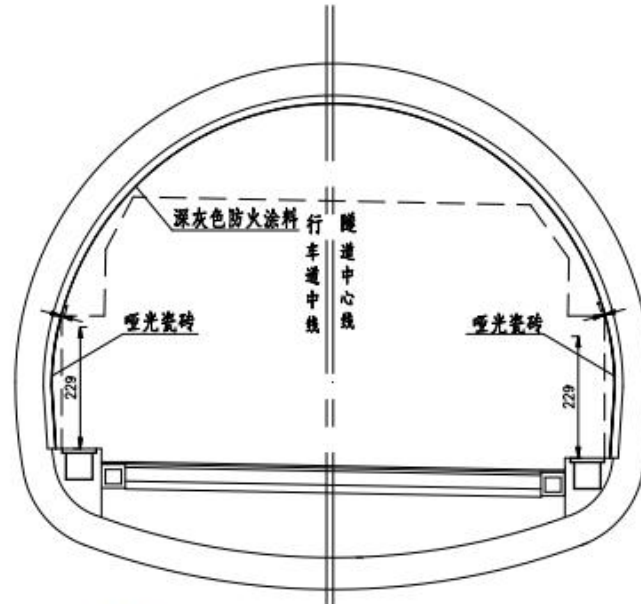
图 6.3-34 隧道内装饰改造设计图（单位：cm）
