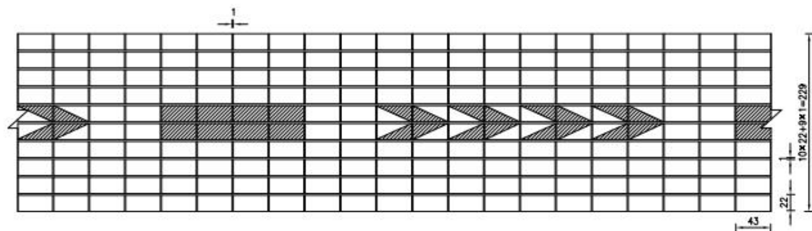
隧道瓷砖铺设设计展开图
